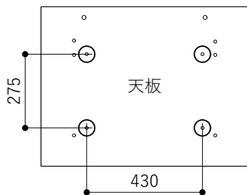
【上面図】
